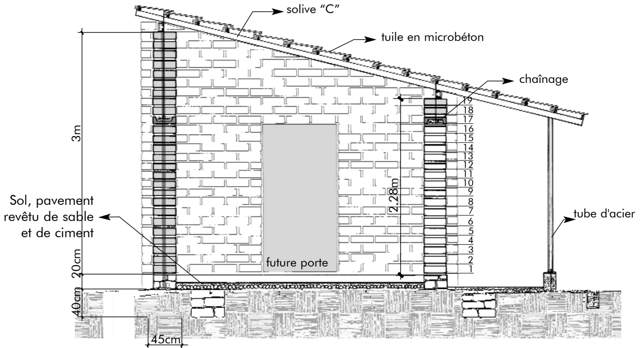
COUPE A-A
