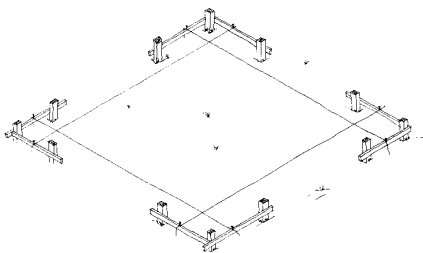
Installation des chaises en bois et des cordes
